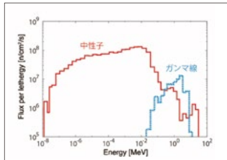
BNCT照射場の中性子とガンマ線スペクトル
