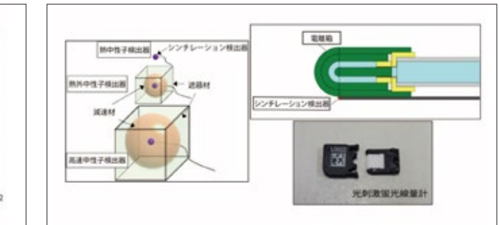
開発した測定システム
