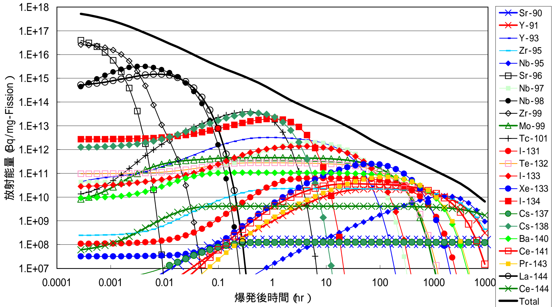
U235核分裂後の FP放射能量 (U235 1mgの fission :1sec ~ 1yr)
