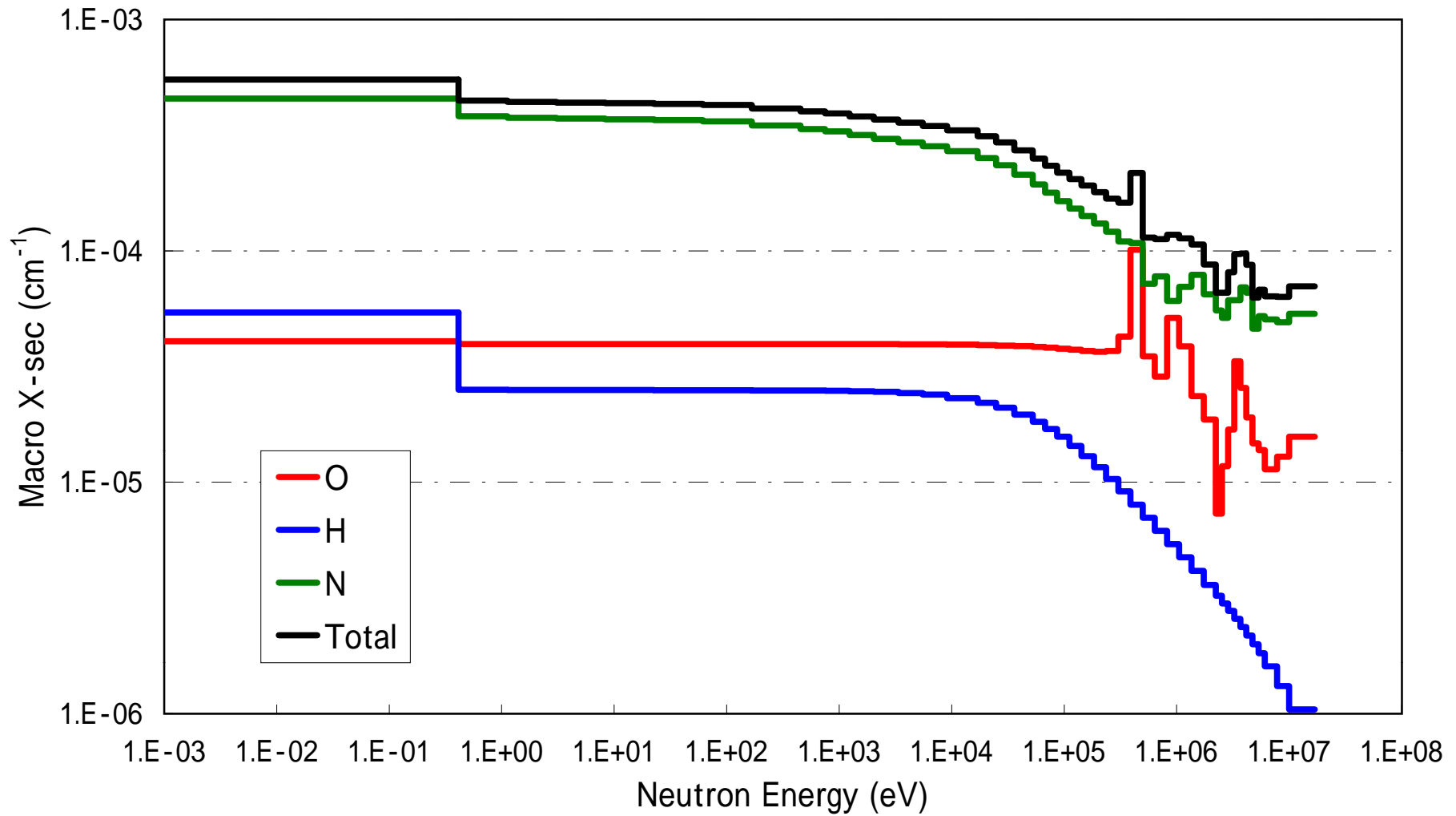
空気の中性子全断面積
