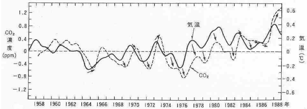
図1 気温の変化と二酸化炭素の変化の対応 CO 2 は気温の上昇より遅れて変化していることがわかる。
