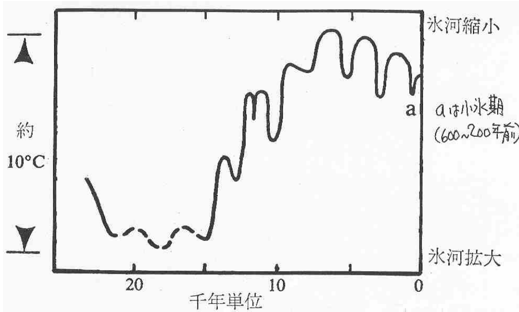
図 3 過去 2 万 5 千年間の北半球の気温の変化
