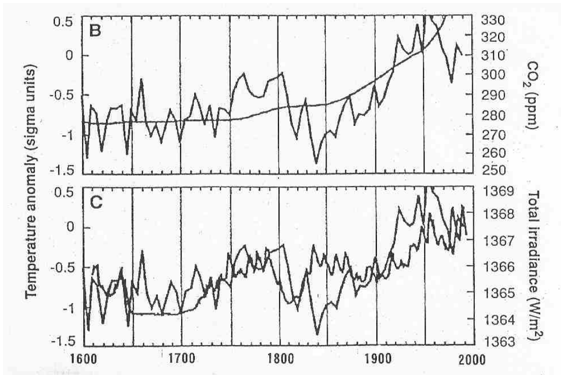
図2 北極圏における気温、CO 2 濃度、照射量の比較
