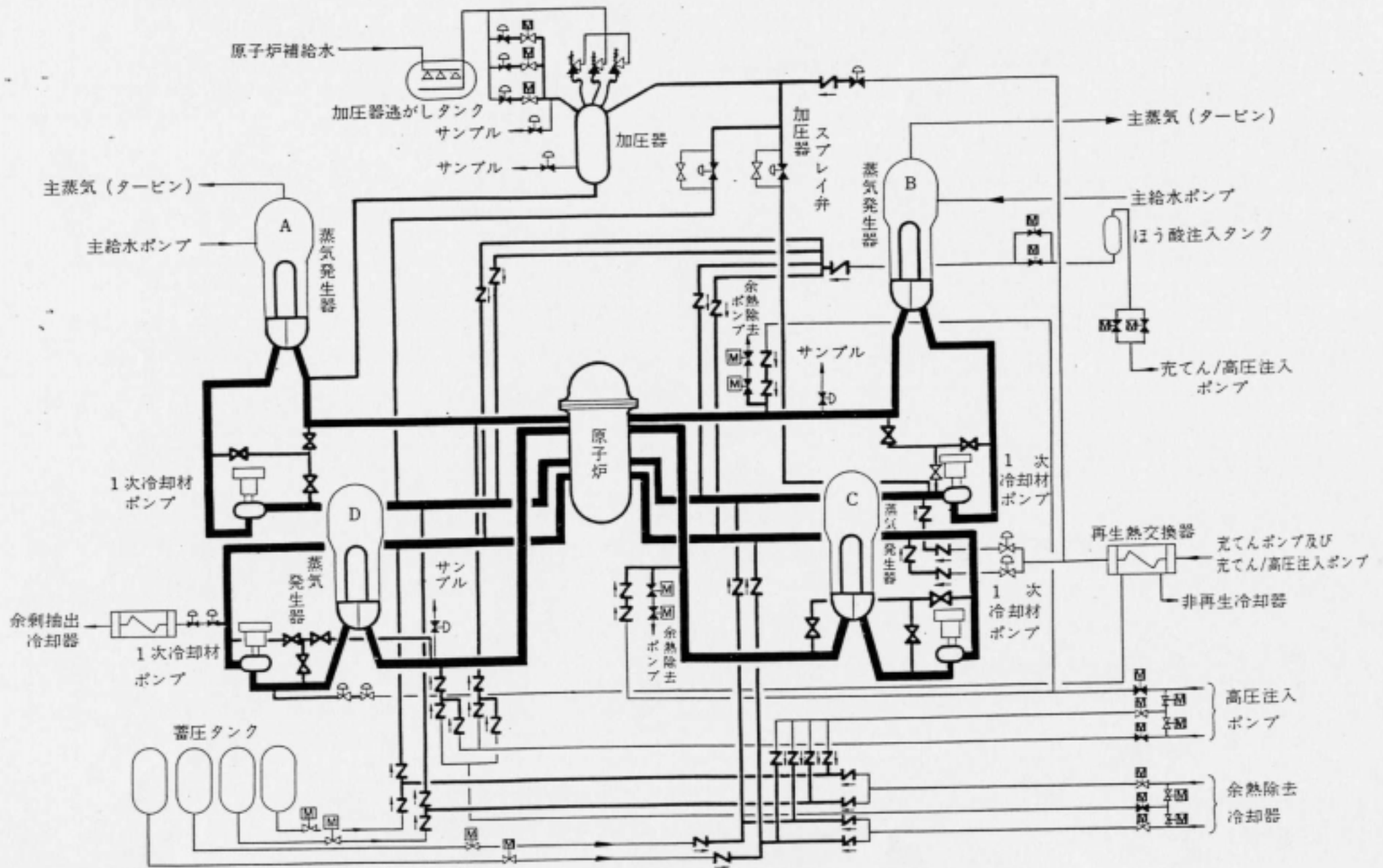
原子炉冷却材圧力バウンダリ説明図
