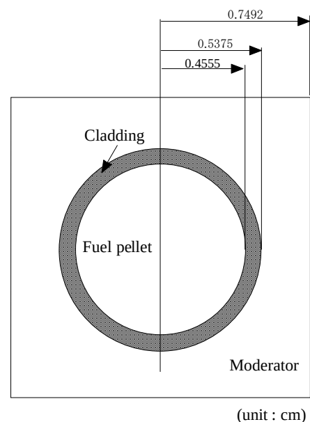
計算体系 (PWR-UO 2 )
