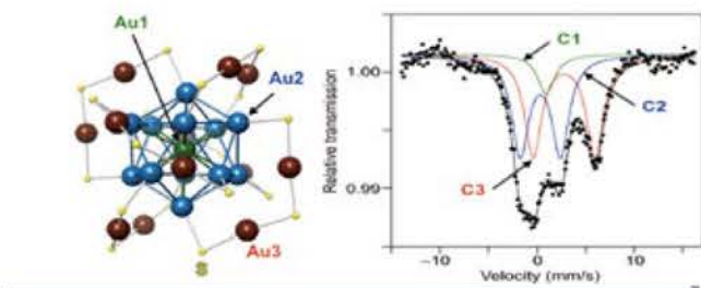
金原子 (Au:色は状態の違いに対応) 25個、硫黄原子 (S) 18個による微粒子 (クラスター) の構造 (左) とその ^{197}\text{Au} メスパウアースペクトル (右)
