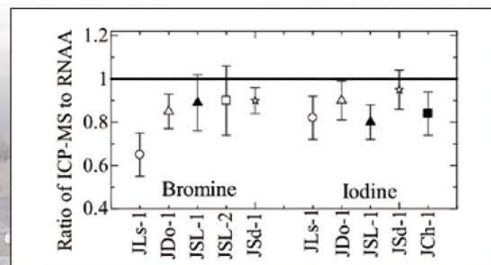
いくつかの堆積岩試料中の臭素とヨウ素の分析値に対して、一般的な元素分析法(ICP-MS)で定量された値が、放射化分析法で定量された値より、系統的に低くなった結果を示している
