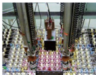
KUCA固体減速架台
