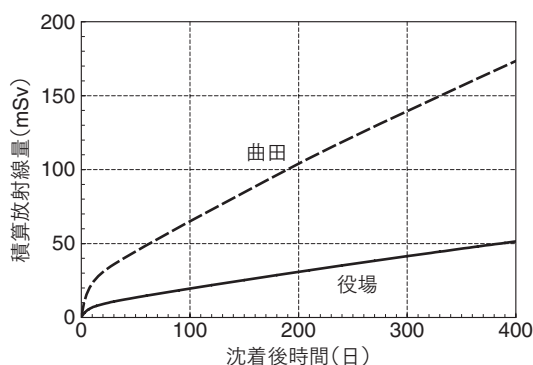
図4—表2の土壤汚染データにもとづく役場と曲田での積算空間線量計算値
