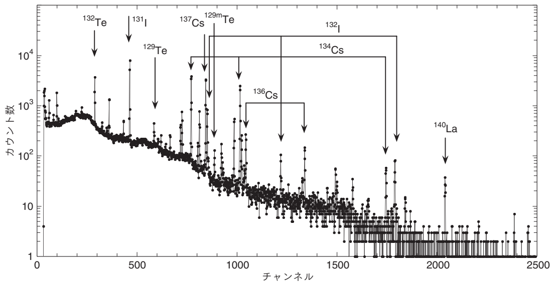
図2—#53で採取した土壌の \gamma 線スペクトル
