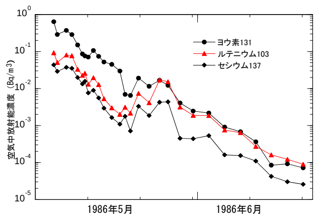
図16. 京大原子炉(大阪府熊取町)で観測した空气中放射能濃度
