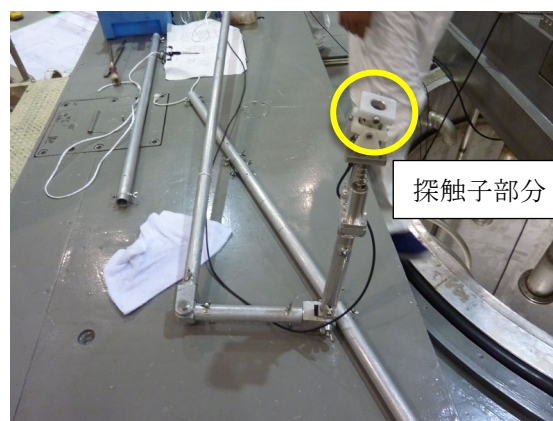
図2 測定治具
