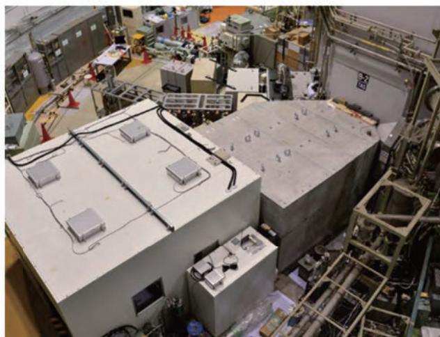
B-2実験孔照射装置
