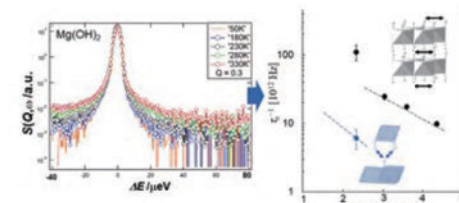
図2: 水酸化マグネシウムの準弾性散乱解析。左側の中性子エネルギー散乱スペクトルの裾部分の幅が、結晶内部の水素跳躍運動の頻度を示す。右側は温度と水素の跳躍頻度の相関図。頻度が異なる二種類の跳躍の経路を発見した。
