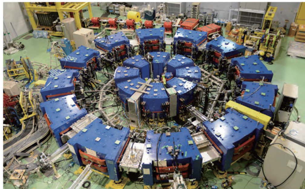
150 MeV FFAG 加速器
