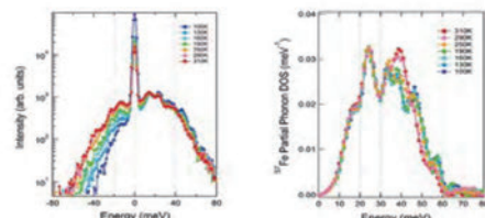
電荷分離酸化物CaFeO 3 の温度変化核共鳴非弾性散乱スペクトル(左)とこれから求めたFeフォノン状態密度(右)。
