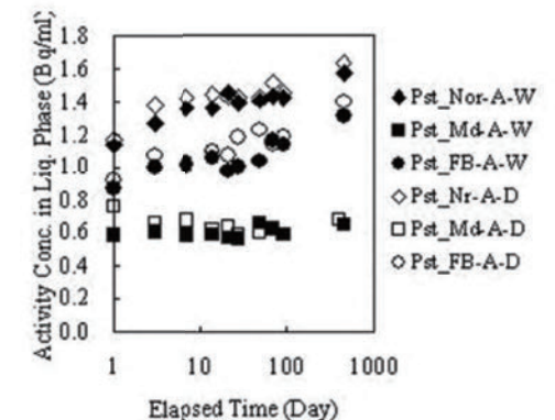
各種セメントからの 137 Csの水中への浸出
