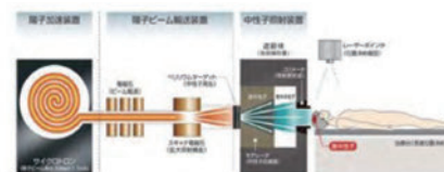
図2 加速器BNCT照射システムのシエマ
