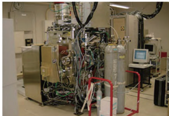
イオンビームスパッタ装置
