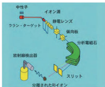
KUR-ISOLの概念図。 ウラン・タングステン中で生成された放射性同位体をキャピラリーを通してイオン源に移送し、イオン化した後、質量分離を行う。
