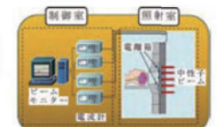
多重電離箱システム
