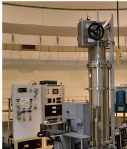
精密制御照射装置(SSS)
