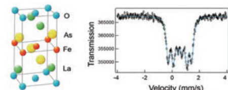
Fe系高温超伝導母物質LaFeAsOの ^{57}\text{Fe} メスバウアースペクトル。
