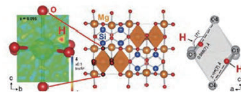
図1: 17万気圧で合成した含水素鉱物「ワスレイト」の構造解析。左側の中性子散乱長分布の赤色(負値)が水素。散乱長から得た水素濃度は1500ppmであり、地球内部でこの結晶が海水の3倍の水素を吸収できることを示した。
