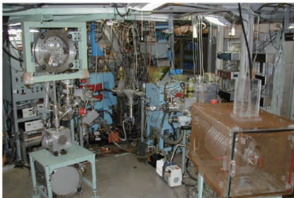
オンライン同位体分離装置(KUR-ISOL)
