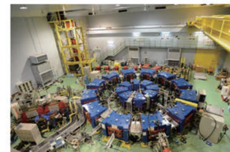
FFAG陽子加速器の全景
