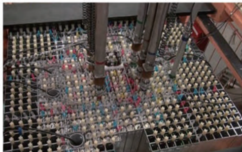
KUCA固体減速架台
