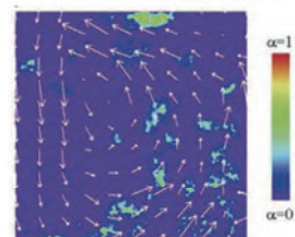
中性子イメージングによって得られた 溶融金属二相流内のボイド率と速度分布
