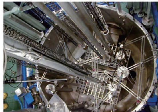
KUCA軽水減速架台
