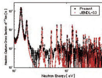
243Amの中性子捕獲断面積
