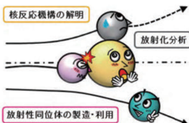
本研究分野の基本となる核反応の概念図
