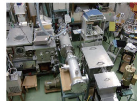
高輝度ミリ波テラヘルツ放射光分光装置
